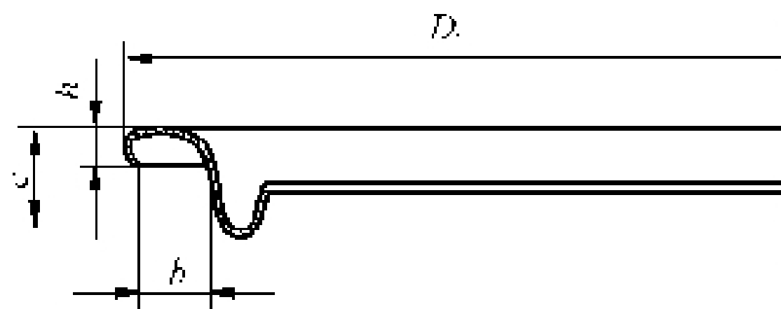
图 5 铝易开盖主要尺寸示意
