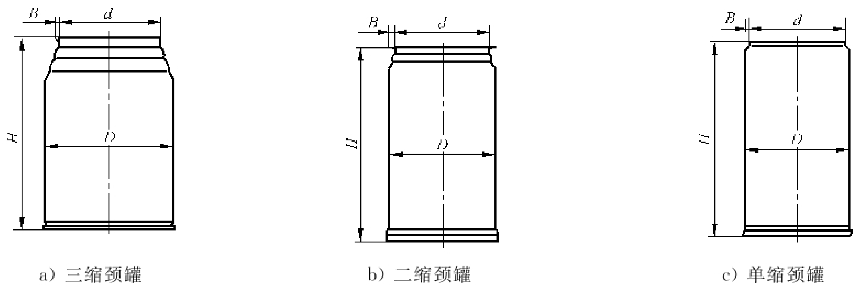
图 1 缩颈罐
