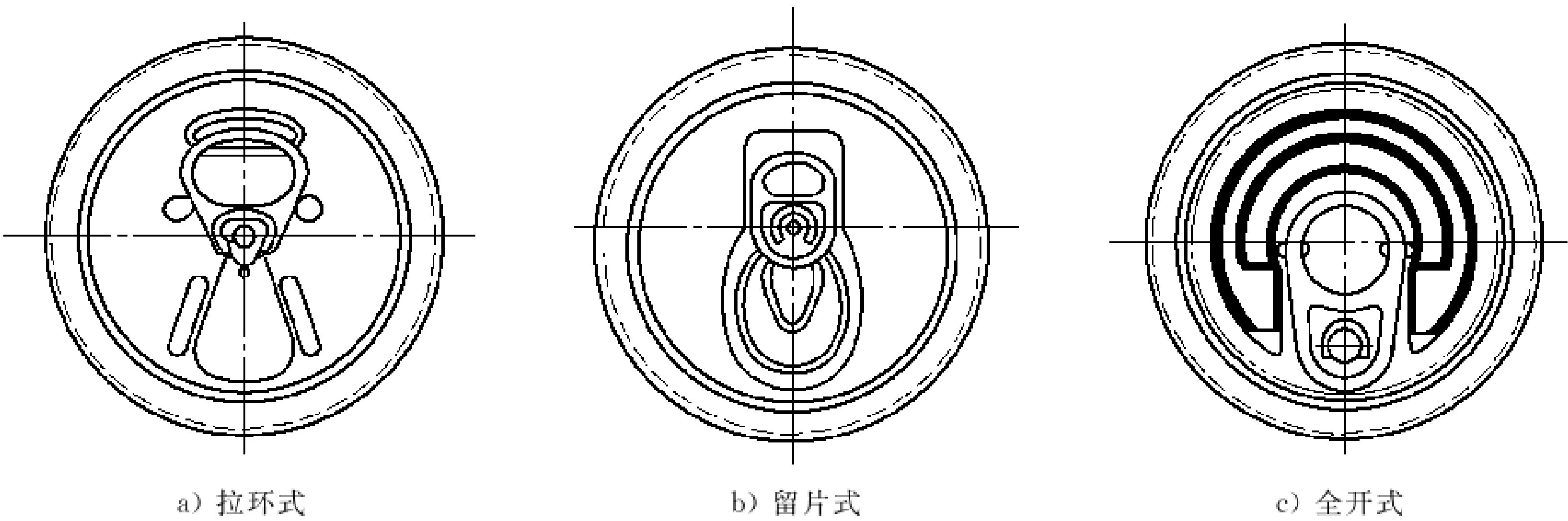
图 3 易开盖
