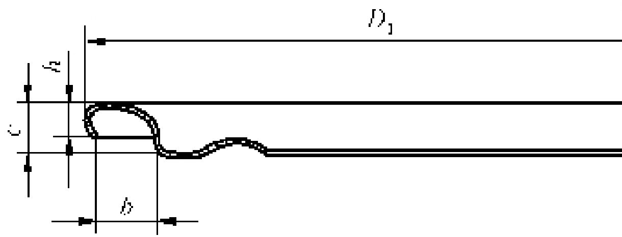
图 6 底盖主要尺寸示意
