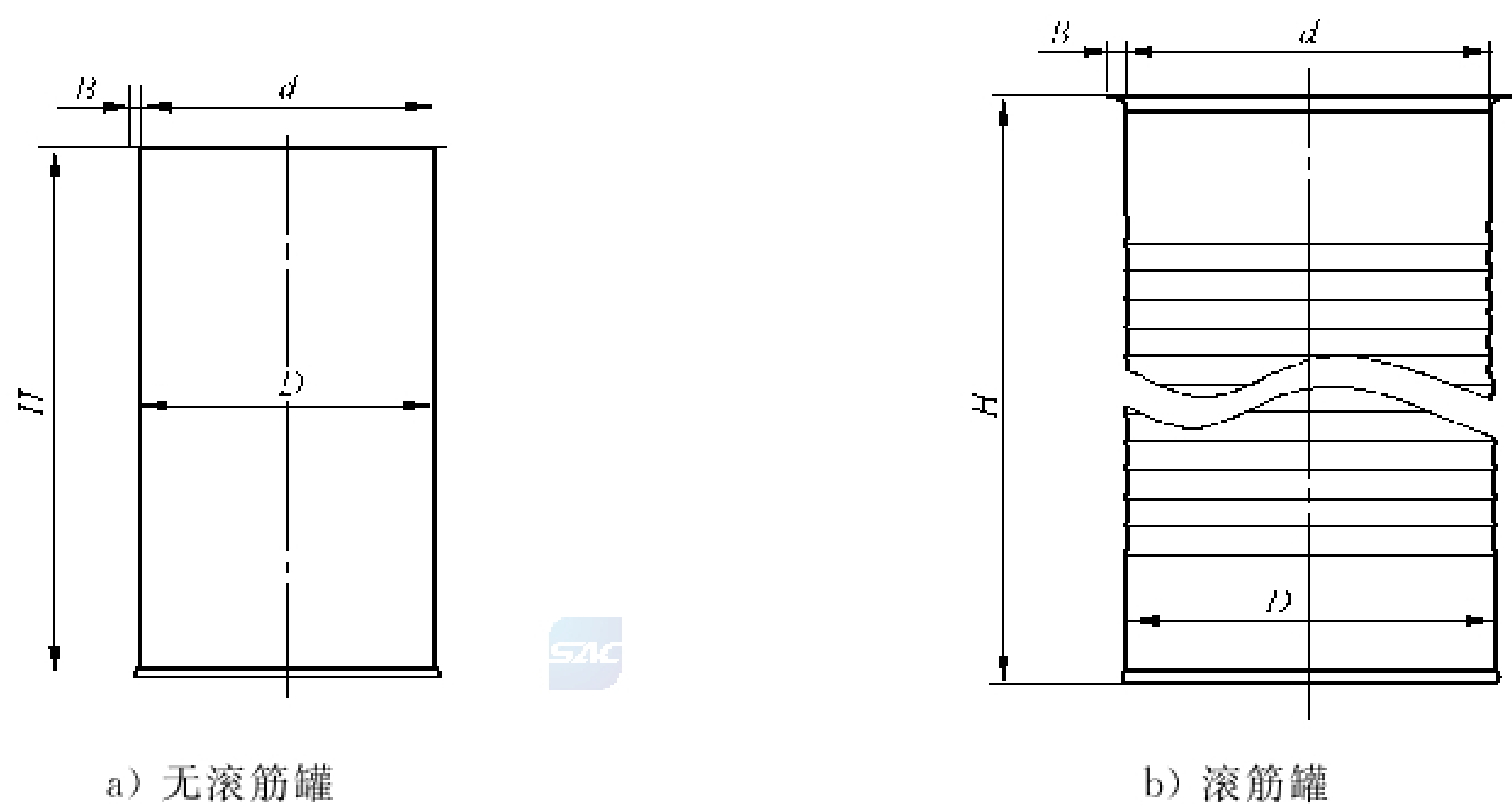
图 2 直身罐
